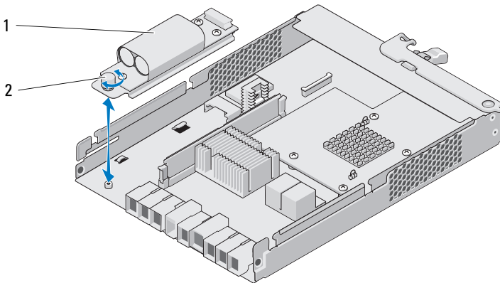
Abbildung 16-10. Entfernen und Installieren des RAID-Controller-Modul-Akkusicherungsmoduls
