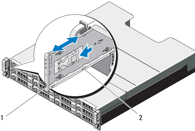
Abbildung 16-13. Entfernen und Installieren der Bedienfeldplatine – PowerVault MD3600i
