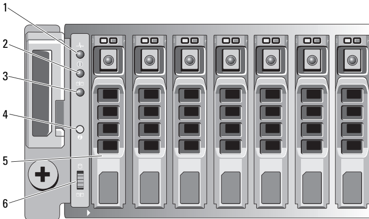
Abbildung 2-2. Funktionen und Anzeigen auf der Vorderseite – Dell PowerVault MD3620i
