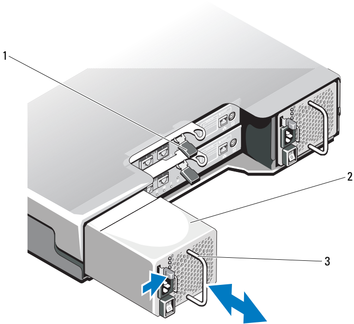
Abbildung 16-11. Entfernen und Installieren eines Netzteil-/Lüftermoduls
