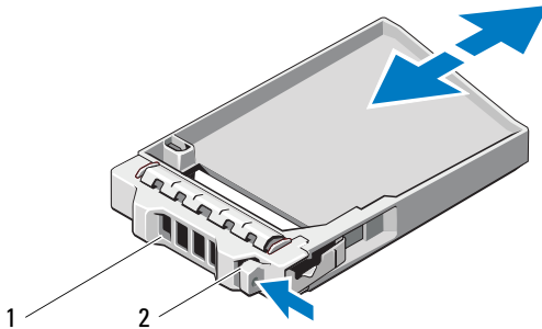
Abbildung 16-3. Entfernen und Installieren eines 2,5-Zoll-Laufwerkplatzhalters (Nur MD3620i)
