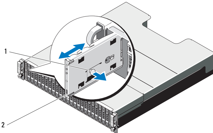
Abbildung 16-14. Entfernen und Installieren der Bedienfeldplatine – PowerVault MD3620i
