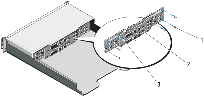
Abbildung 16-16. Entfernen und Installieren der Rückwandplatine – PowerVault MD3600i
